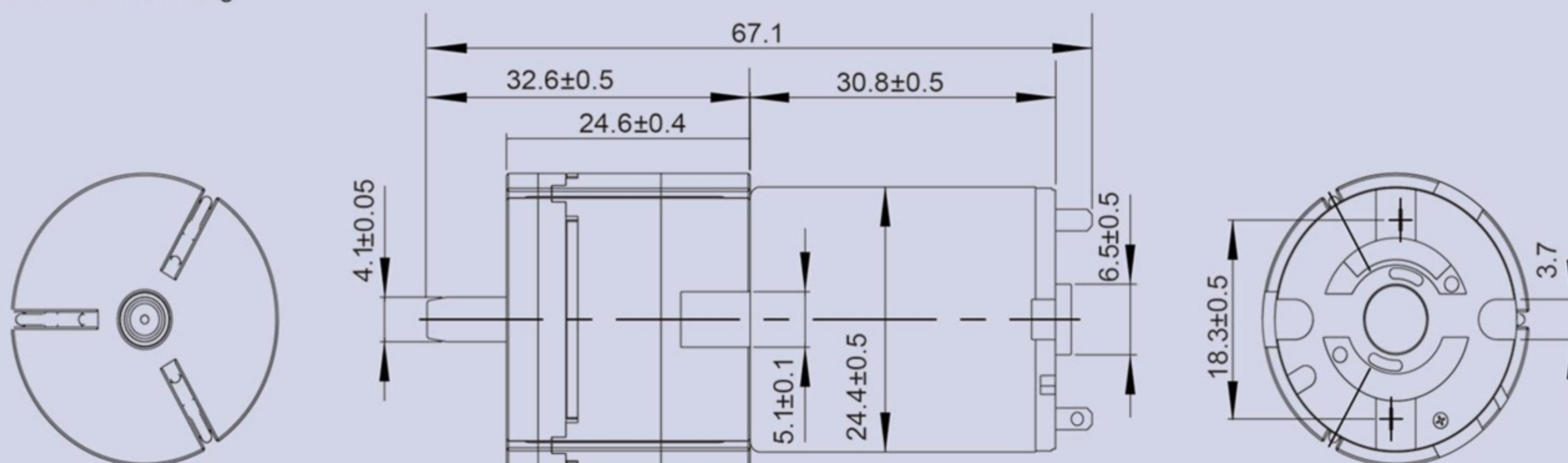
產品構造圖 Dimension Drawing
