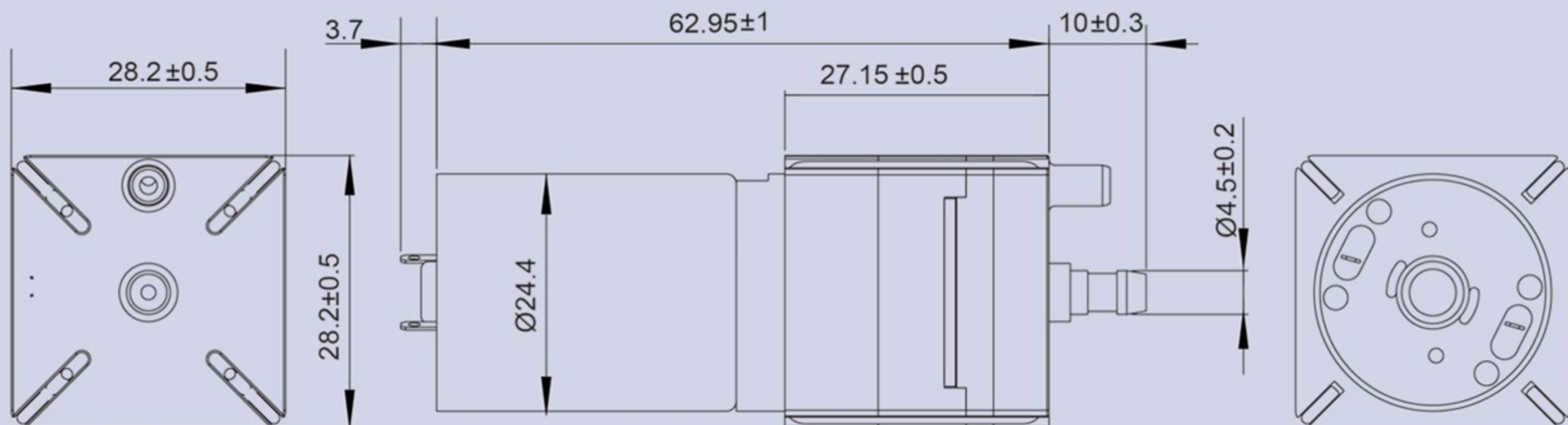
產品構造圖 Dimension Drawing
