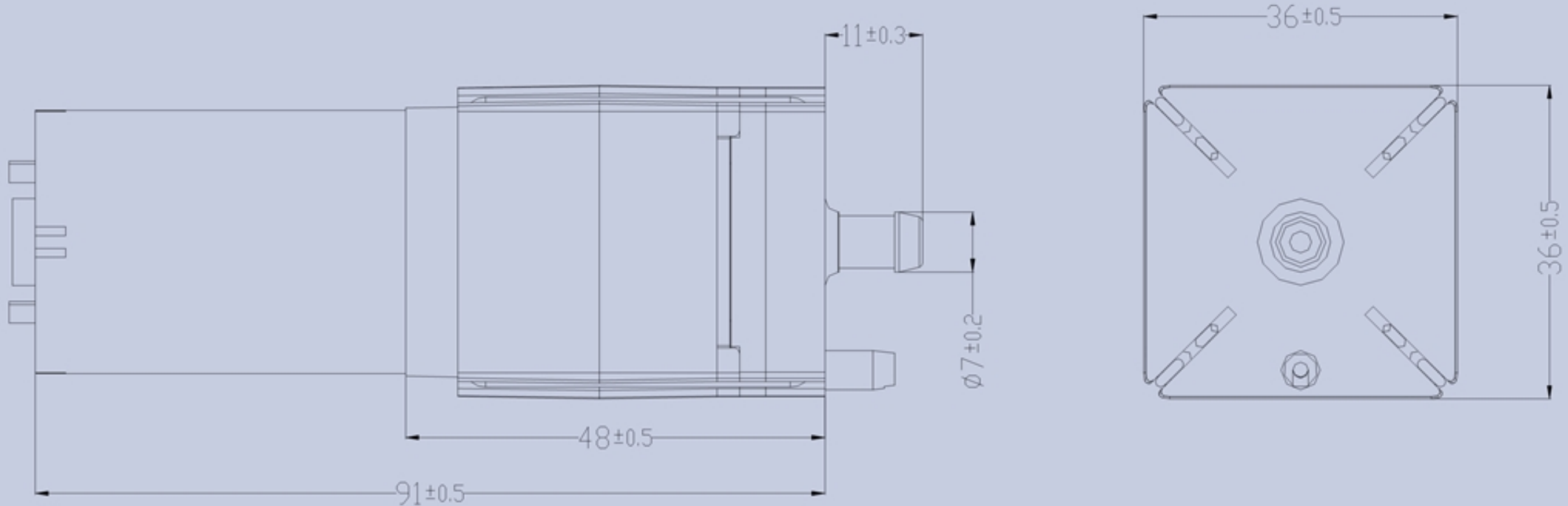
產品構造圖 Dimension Drawing
