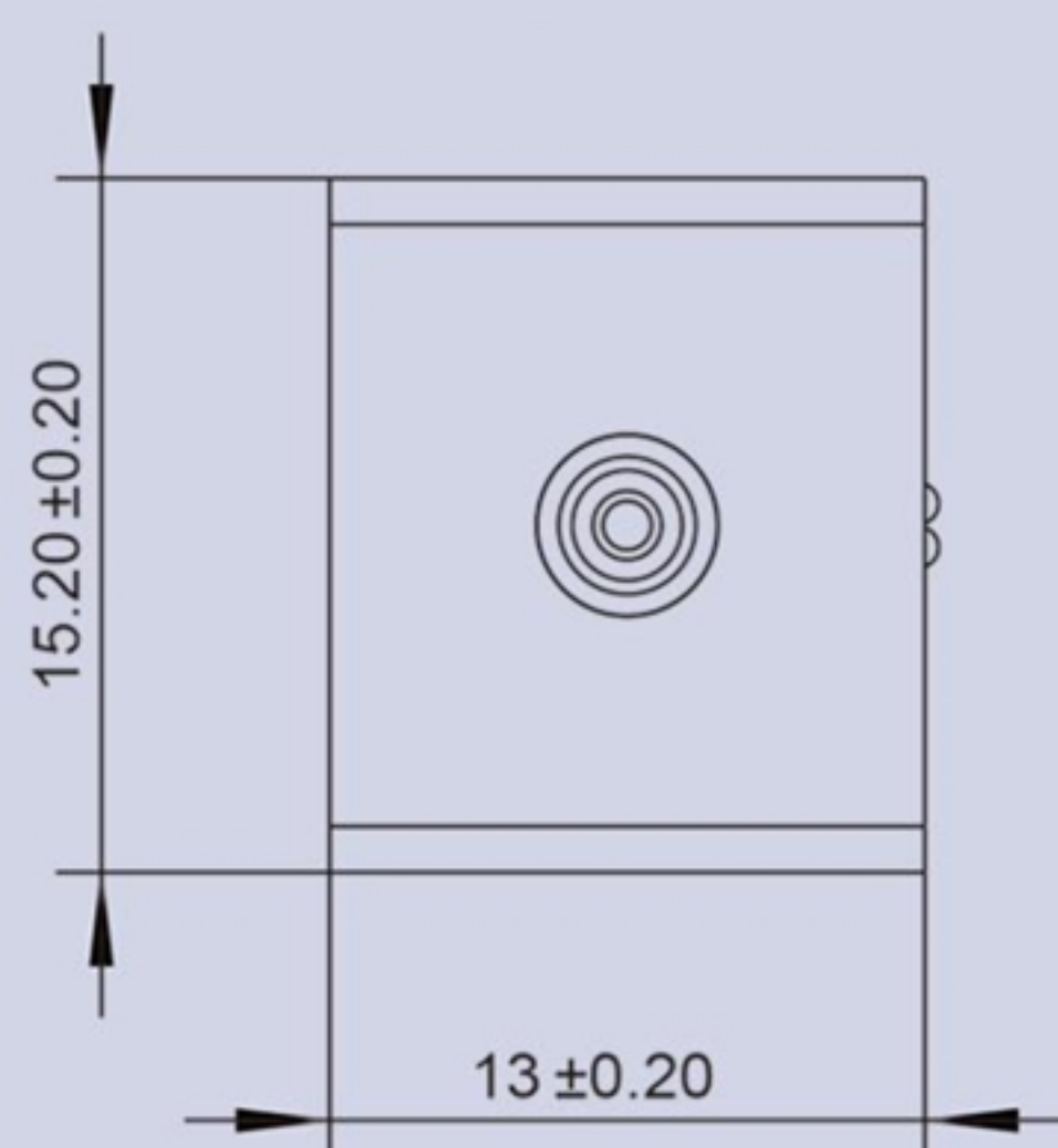
產品構造圖 Dimension Drawing
