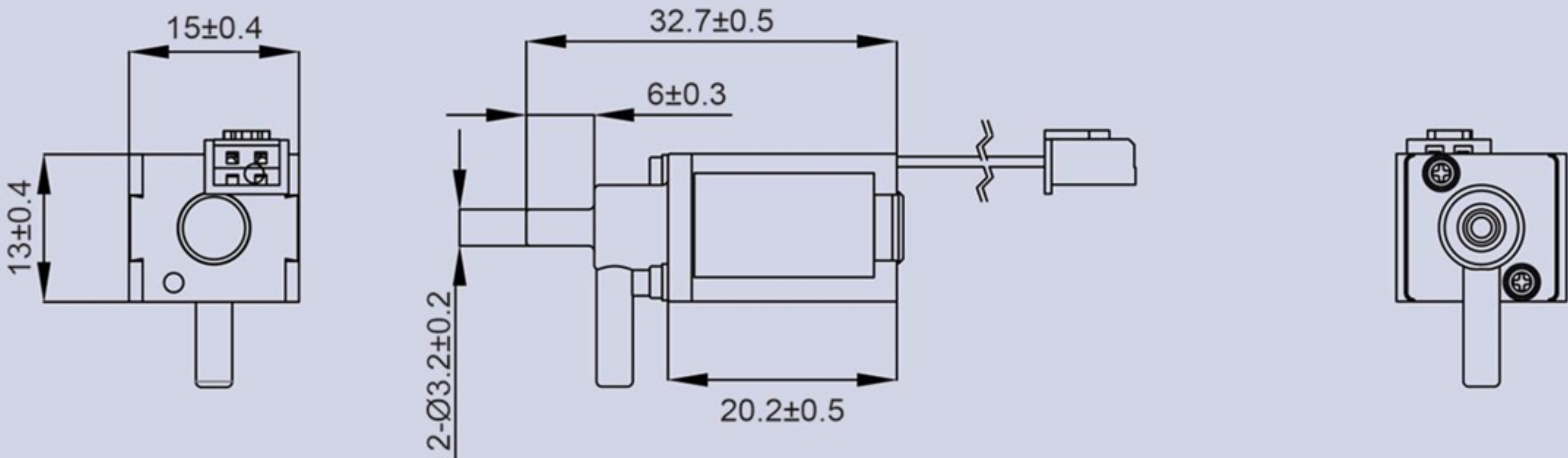
產品構造圖 Dimension Drawing
