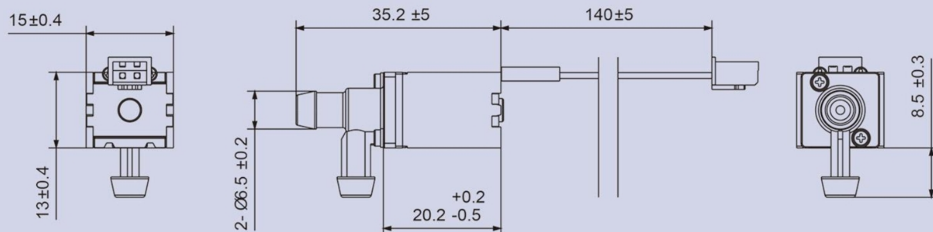
產品構造圖 Dimension Drawing
