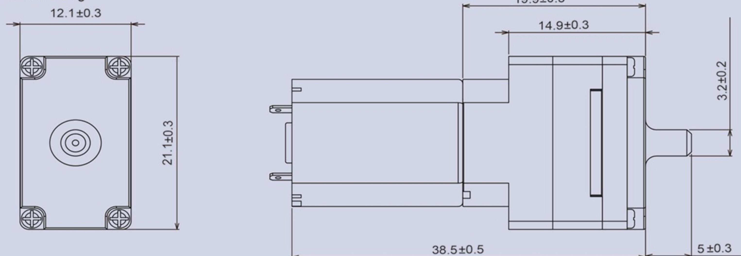
產品構造圖 Dimension Drawing
