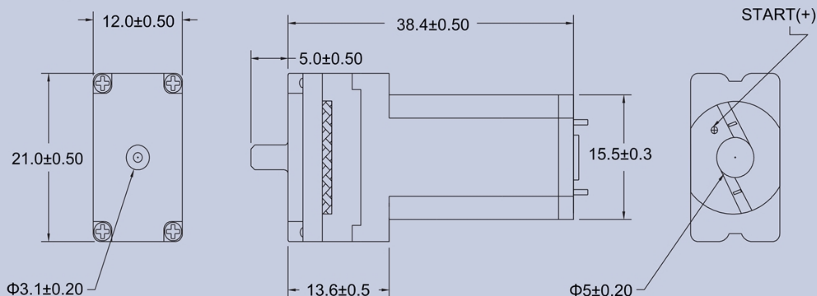
產品構造圖 Dimension Drawing
