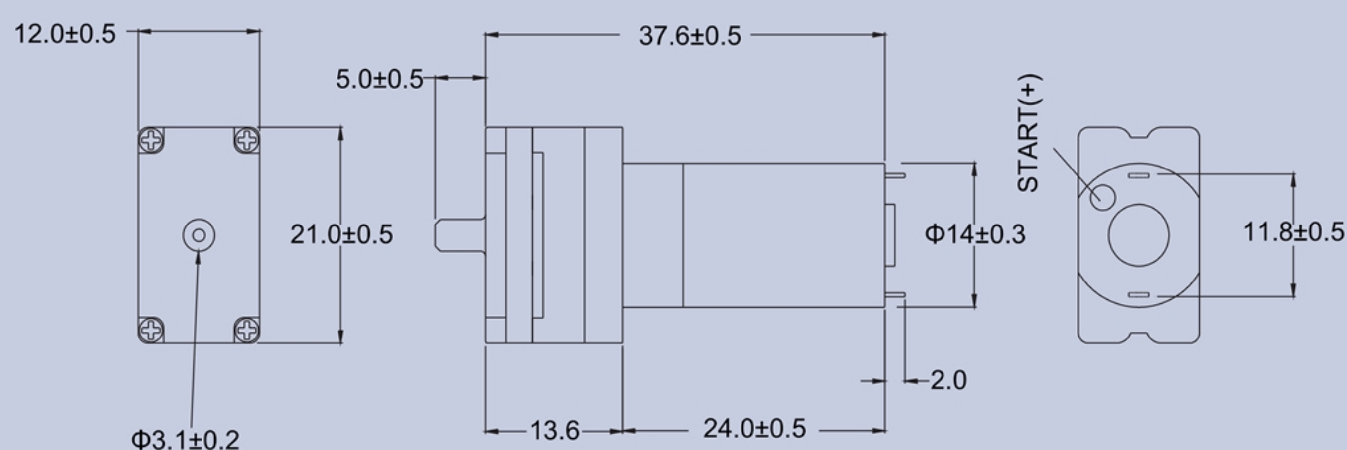
產品構造圖 Dimension Drawing
