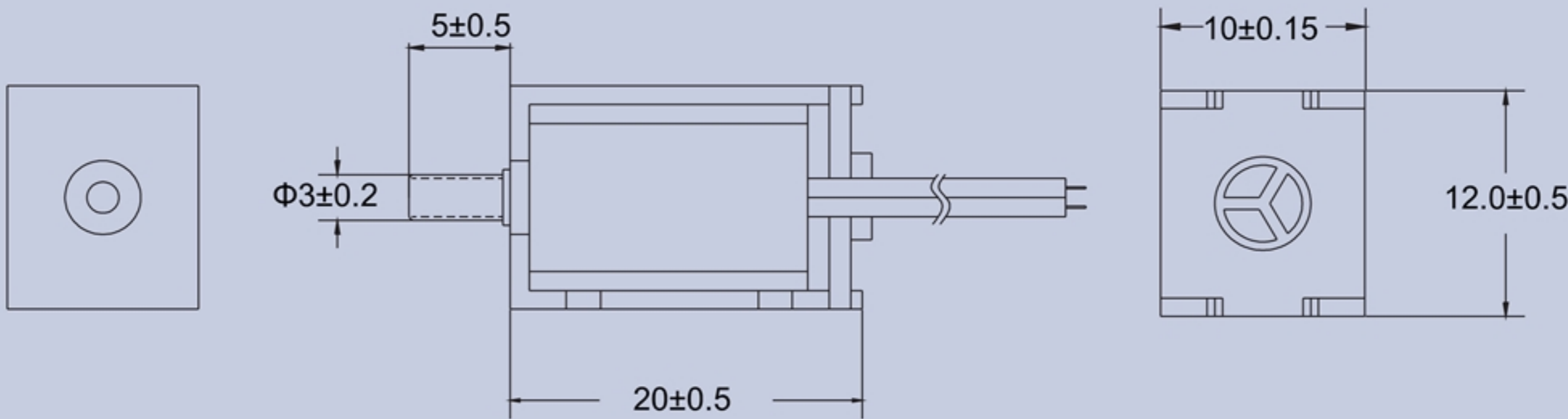
產品構造圖 Dimension Drawing
