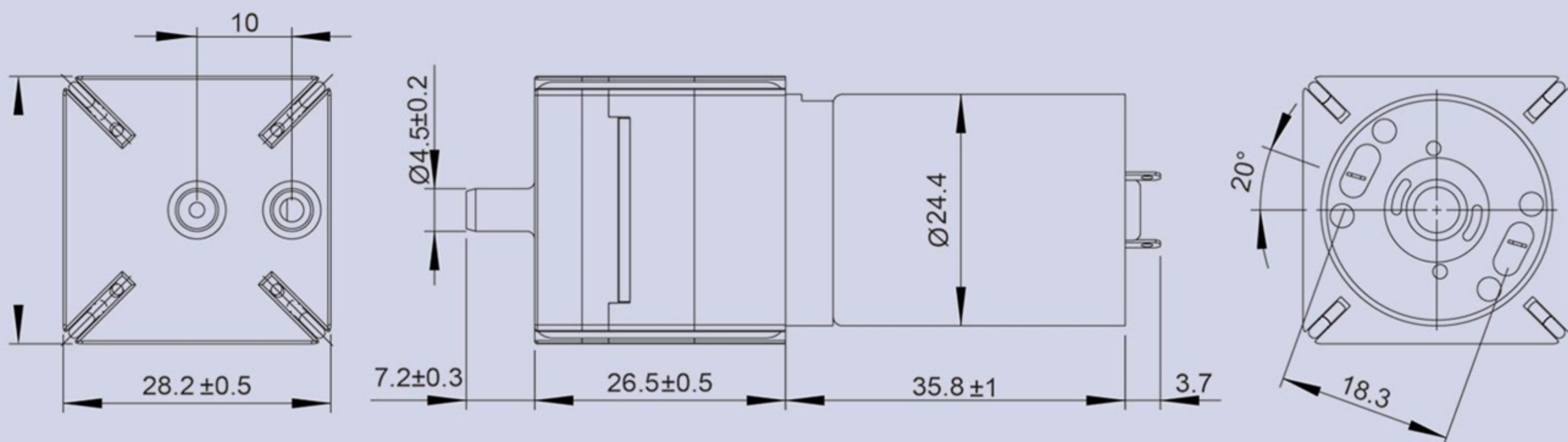
產品構造圖 Dimension Drawing
