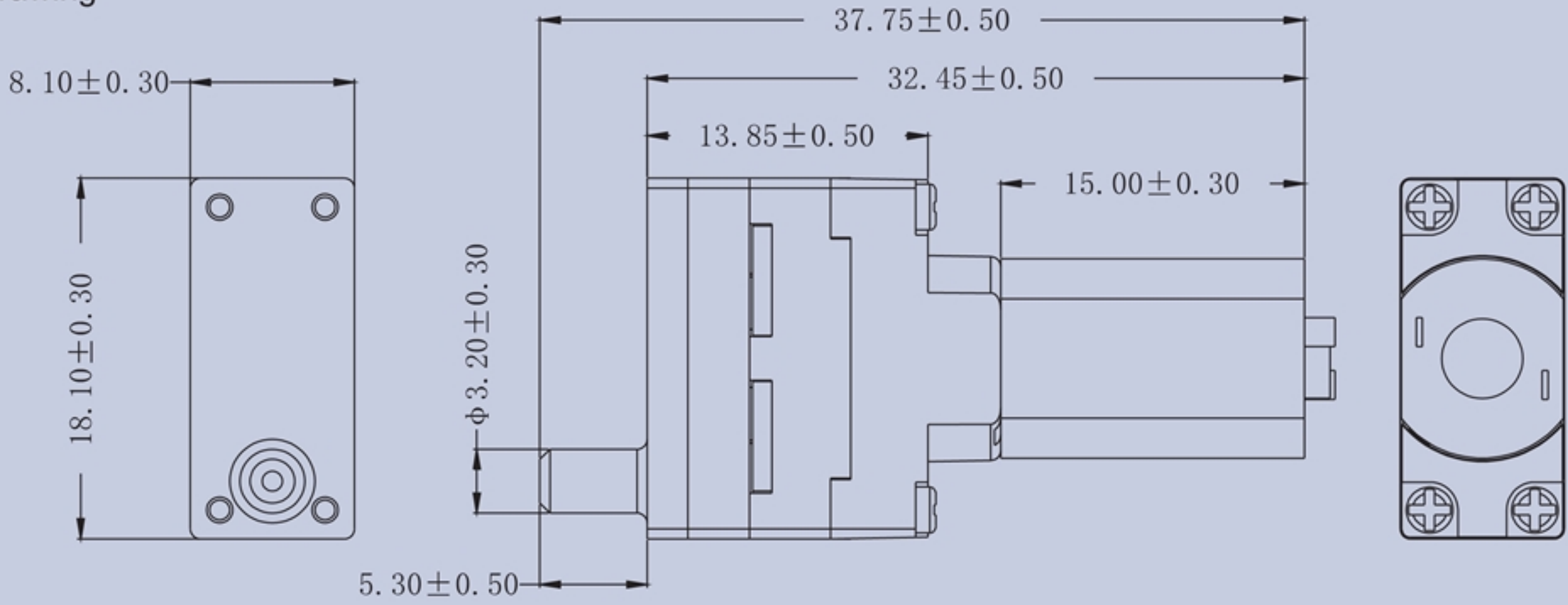
產品構造圖 Dimension Drawing
