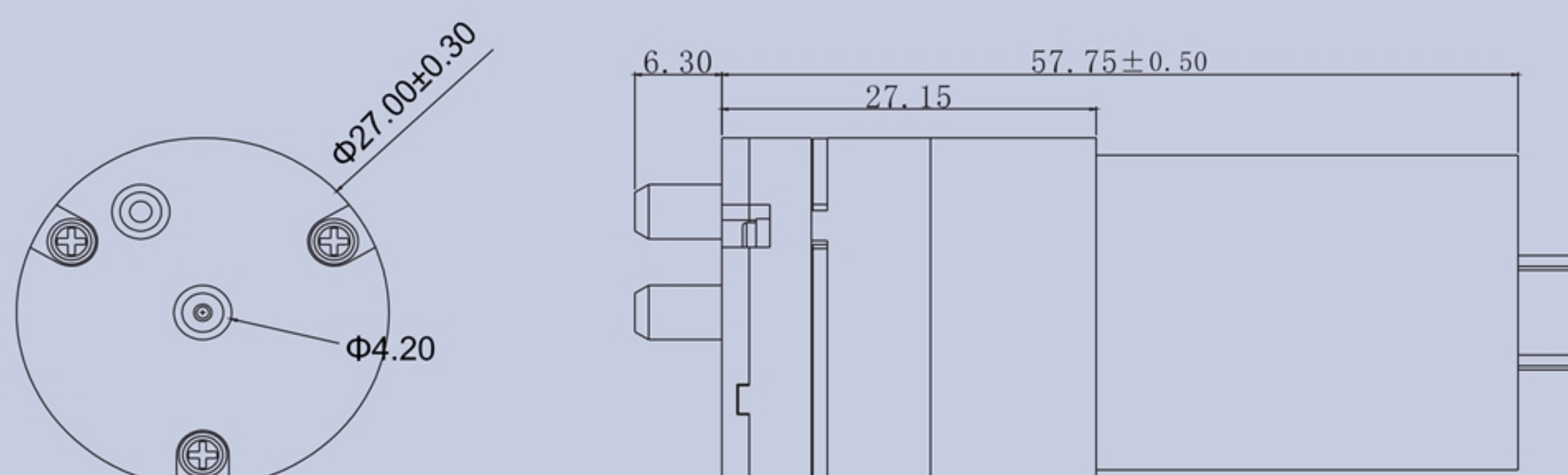
產品構造圖 Dimension Drawing
