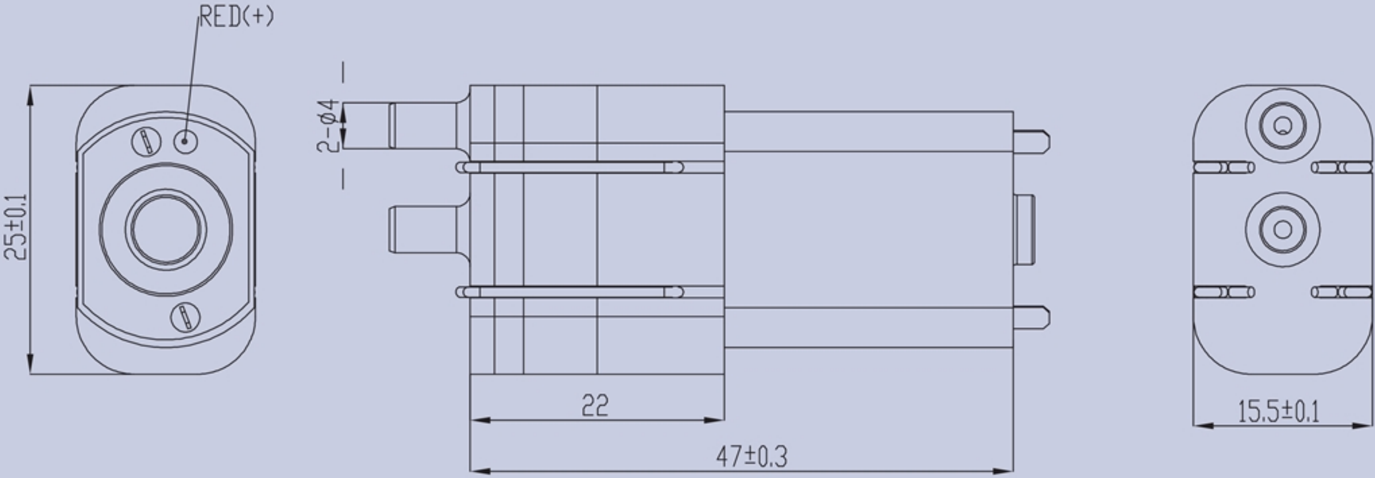
產品構造圖 Dimension Drawing
