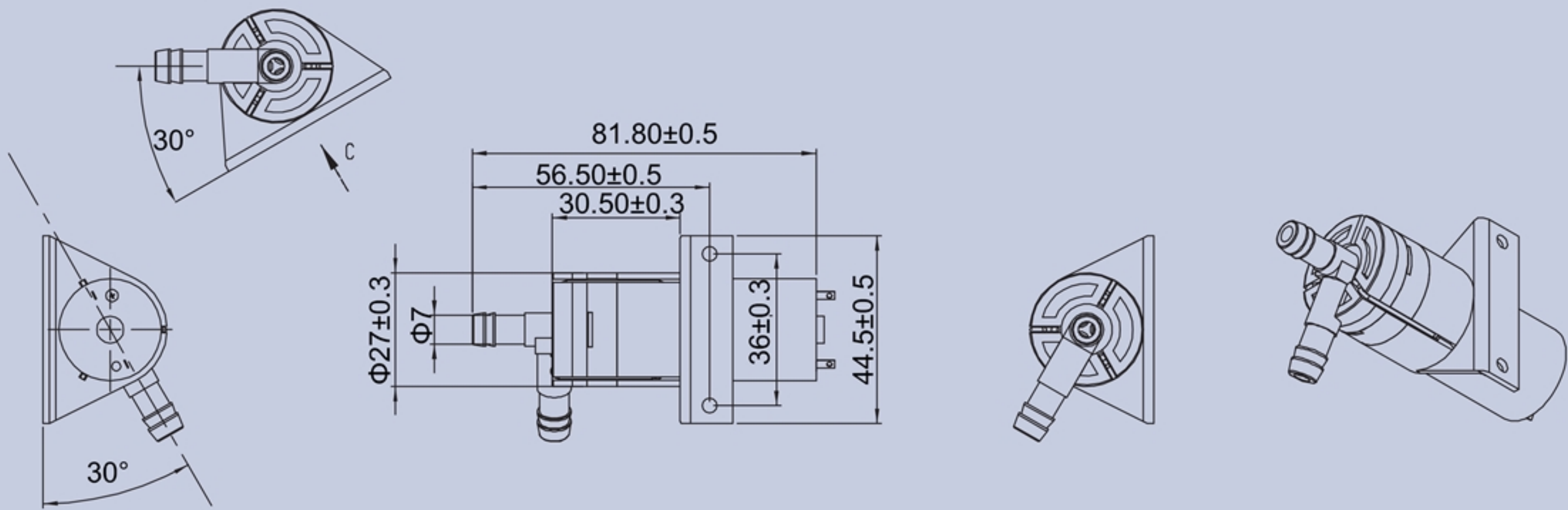
產品構造圖 Dimension Drawing
