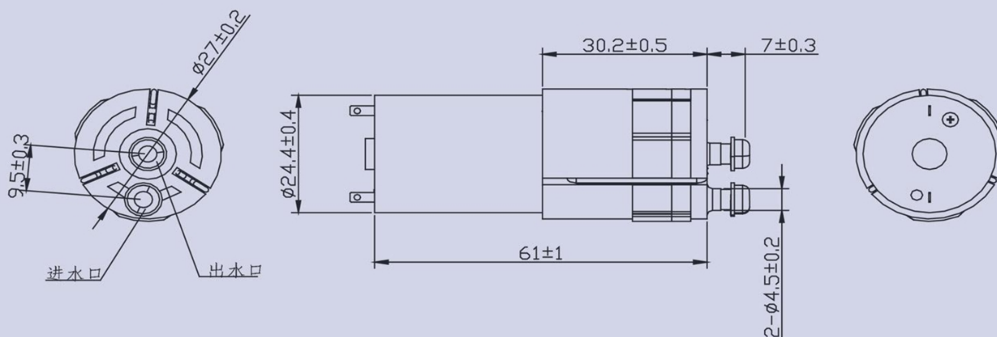
產品構造圖 Dimension Drawing
