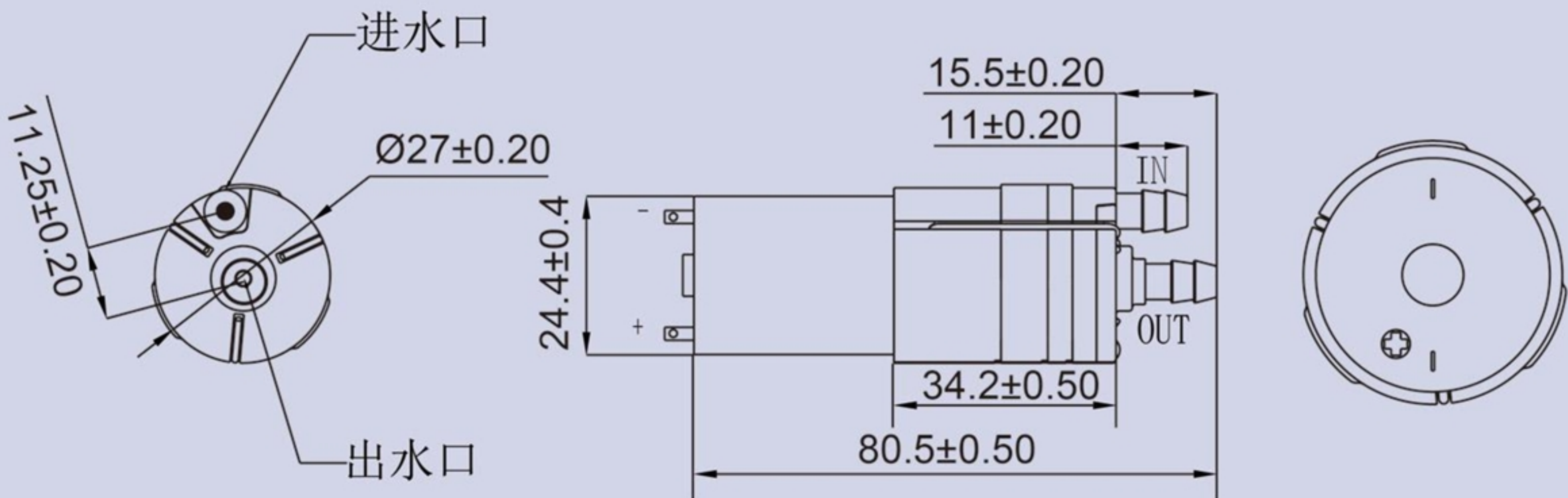
產品構造圖 Dimension Drawing
