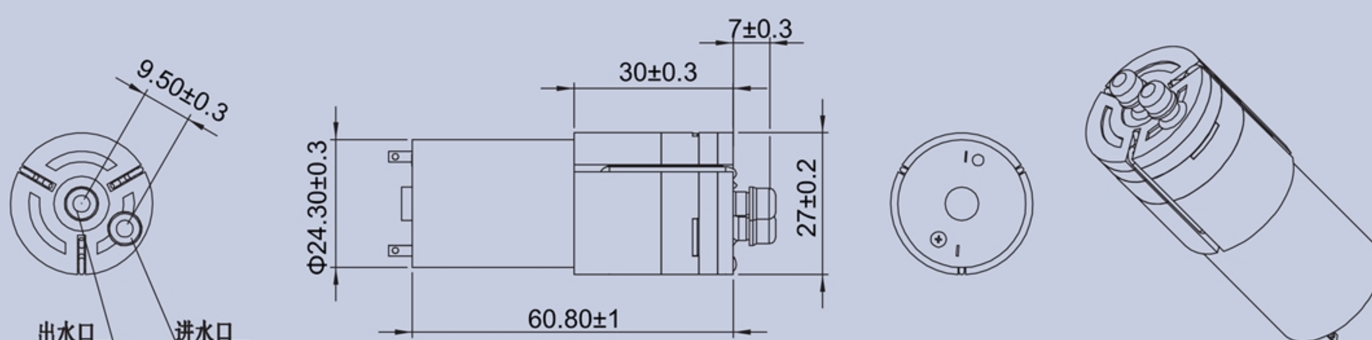
產品構造圖 Dimension Drawing
