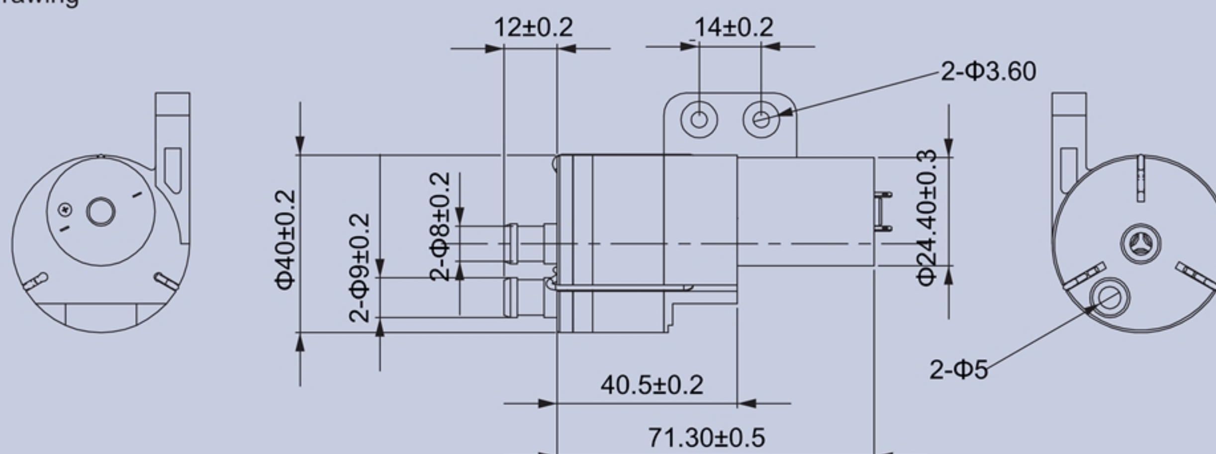
產品構造圖 Dimension Drawing
