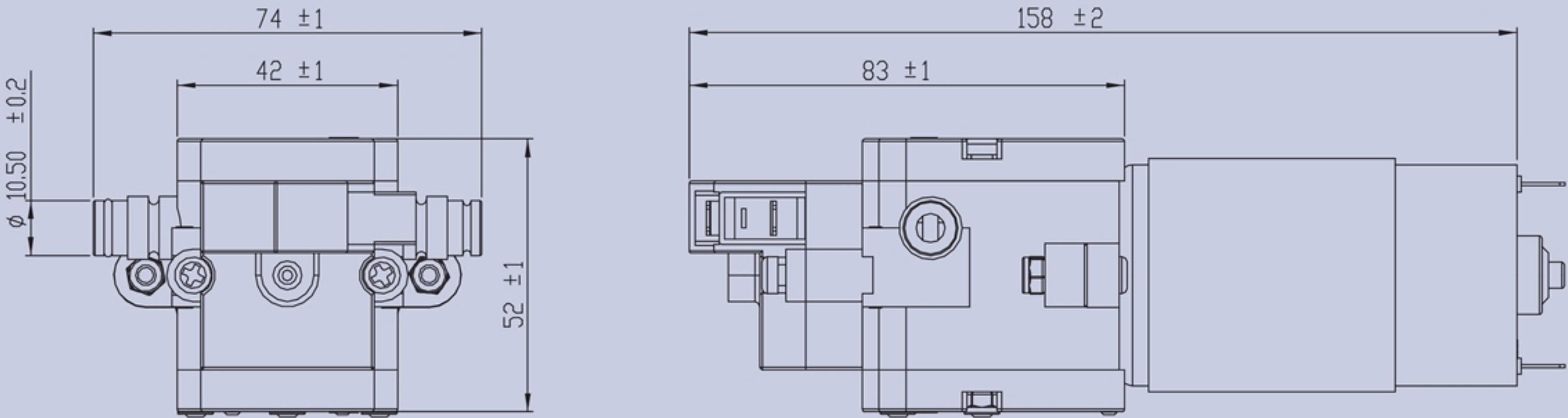
產品構造圖 Dimension Drawing
